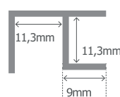
100. Flächenbündige Ecke
