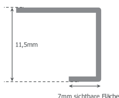
C. – Abschlussprofil
