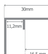
101. Unsichtbare Ecke
